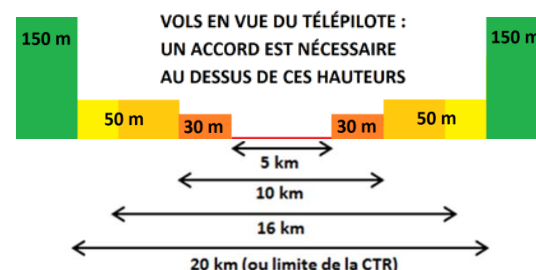
Vues transversales
