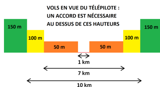
Vue transversale
